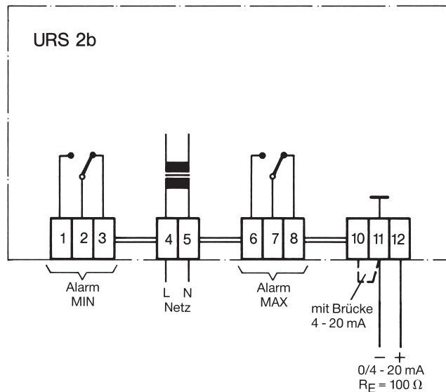
Anschlussplan Grenzwertschalter URS 2b, gezeichnete Kontaktstellungen: stromlos bzw. Alarm
