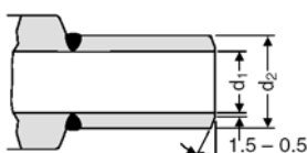
Kończówki do spawania (UNA 16)
