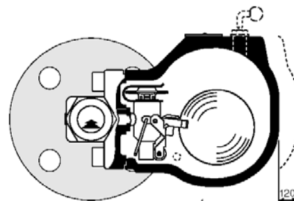
UNA 14h / UNA 16h (pozioma) Wykonanie Duplex
