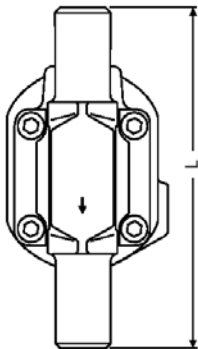
UNA 16v końcówki do spawania
