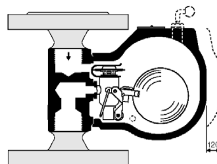
UNA 14v / UNA 16v (pionowa) Wykonanie Duplex
