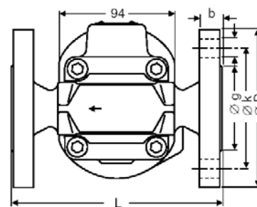
UNA 14h/UNA 16h wersja kołnierzowa
