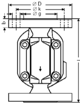
UNA 14v/UNA 16v wersja kołnierzowa
